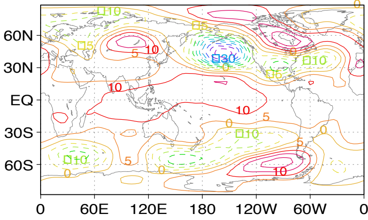
ncep eof1 gh djf
