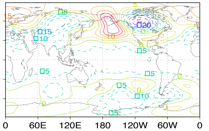
gh alb 0.28 109 djf
