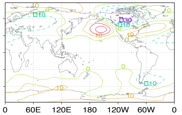
gh alb 0.28 105 djf
