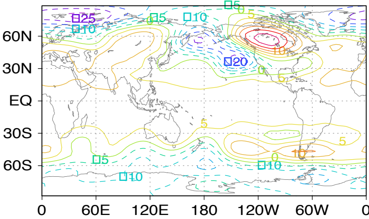
gh alb 0.28 103 djf
