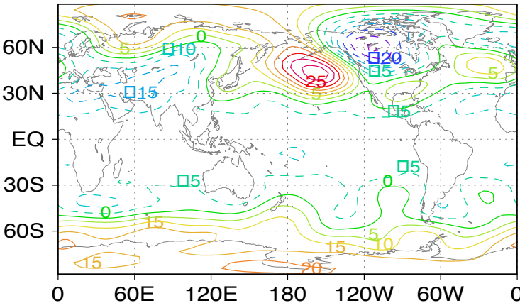
gh alb 0.28 101 djf
