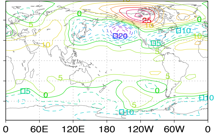
gh alb 0.28 107 djf
